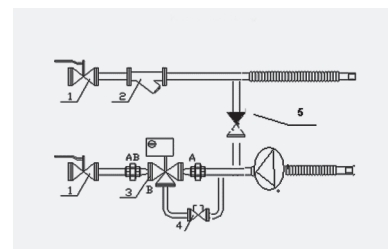
Схема узла терморегулирования Исполнение 3
