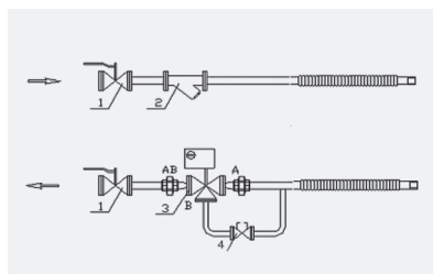
Схема узла терморегулирования Исполнение 1
