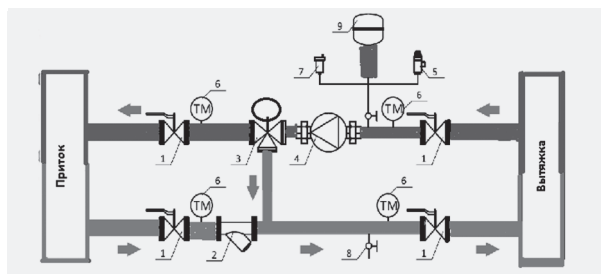
Схема узла терморегулирования для гликолевых рекуператоров SUS-P
