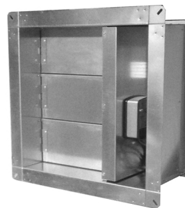
Клапан КДМ-3-ЛС с электромеханическим приводом
